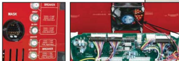
Fan Assembly
